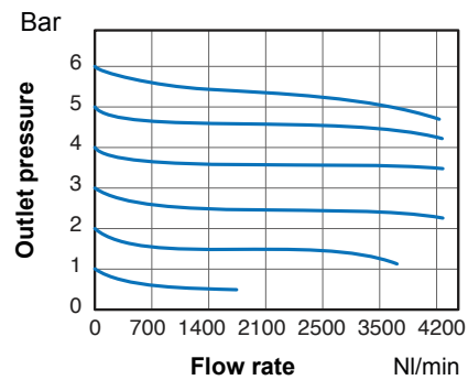
FLOW CHART FPRP04 / FPRPG04
