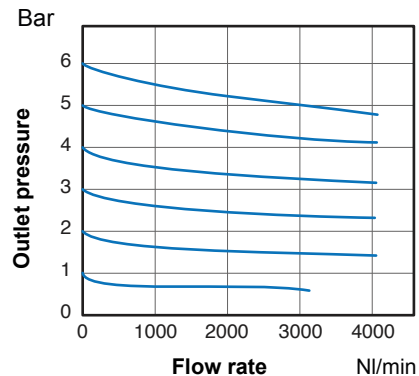
FLOW CHART FPFRM04 / FPRMG04
